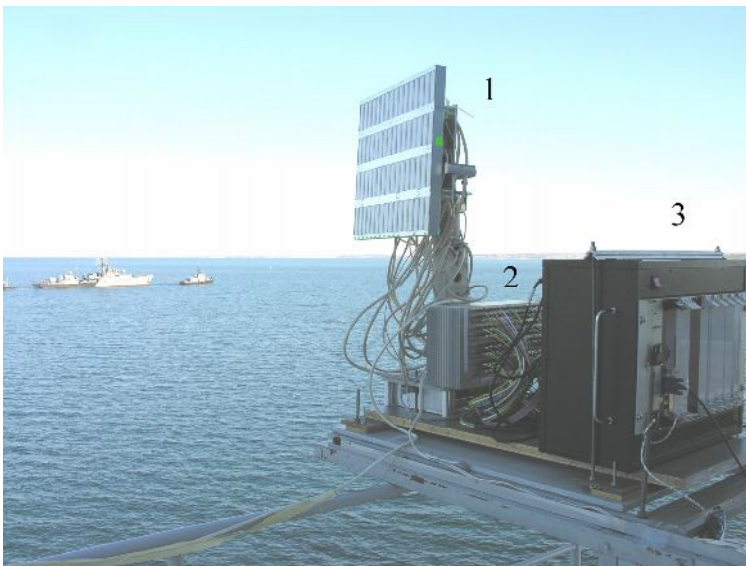
Рис. 9. Приймальний сегмент РЛС
