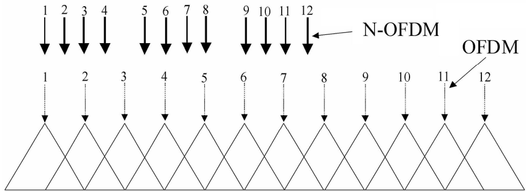
Рис. 3. Компонування N-OFDM (OFDM) сигналу.
